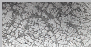
フローフォーミング前の鋳造素材断面
